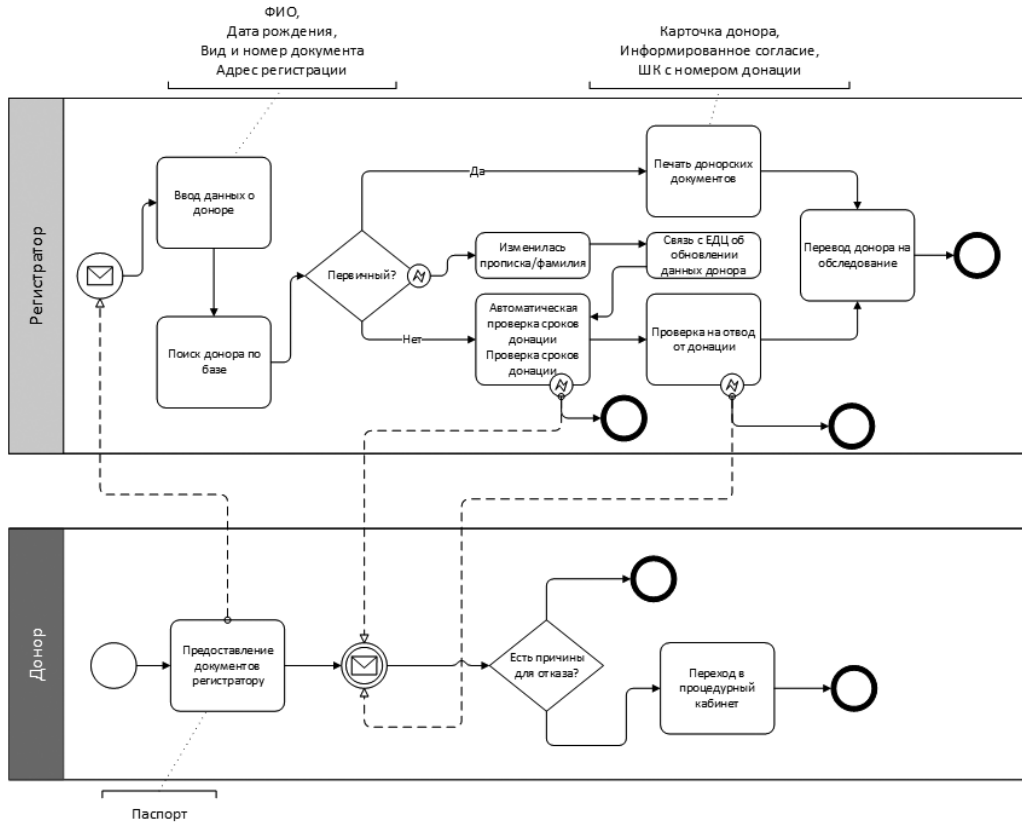
Рис. 3. АРМ «Регистратор».
